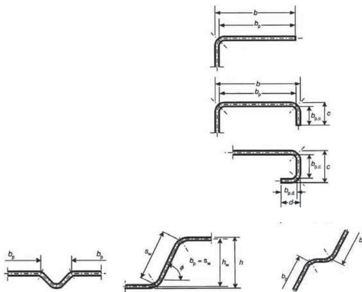
Figura C4.2.27 – Esempi di determinazione della larghezza b_p
