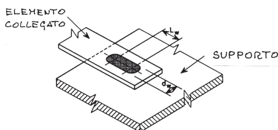
Figura C4.2.36 – Saldature oblunghie a bottone
