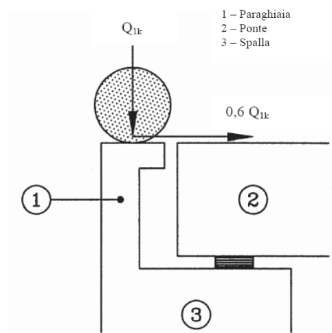
Figura C5.1.1 Carichi da traffico su muri paraghiaia
