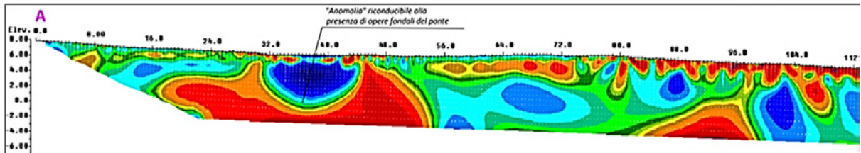
Figura 6 -Sezione tomografica elettrica con evidenza dell' arco rovescio di fondazione dell'antico ponte romano sul Busento antico.
